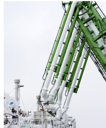
Unloading arms in Montoir de Bretagne, France
