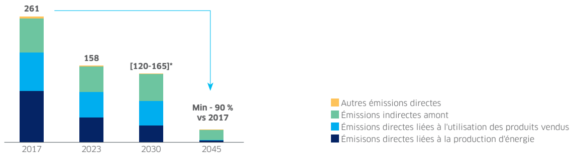
ÉVOLUTION DES ÉMISSIONS D'ENGIE À 2045 (MT CO 2 ÉQ.)
