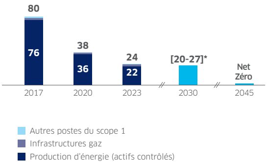
ÉMISSIONS DIRECTES DE GES DU SCOPE 1 (Mt CO 2 équ.)
