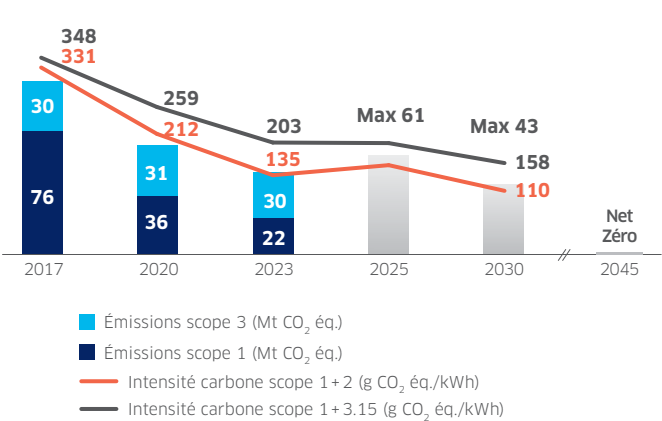
ÉMISSIONS DIRECTES DE GES DU SCOPE 1 (Mt CO 2 équ.)
