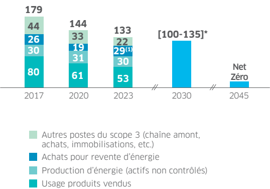
ÉMISSIONS INDIRECTES DE GES DU SCOPE 3 (Mt CO 2 équ.)
