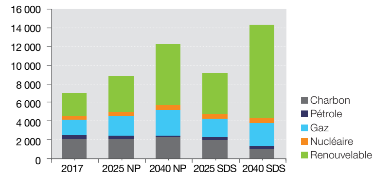
PRÉVISIONS DE CAPACITÉS ÉLECTRIQUES PAR SOURCE DANS LES SCÉNARIOS DE L'AIE (GW)
