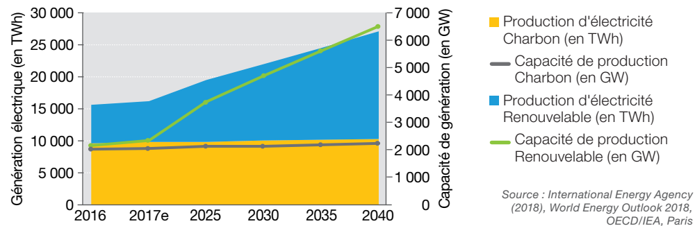
ÉVOLUTION DES CAPACITÉS ET DES PRODUCTIONS ÉLECTRIQUES DANS LE MONDE (NEW POLICIES SCENARIO)
