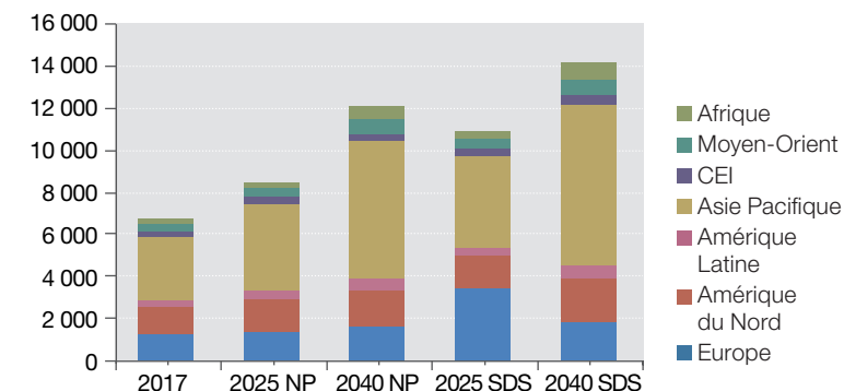
PRÉVISIONS DE CAPACITÉS ÉLECTRIQUES PAR RÉGION DANS LES SCÉNARIOS NEW POLICIES ET SUSTAINABLE DEVELOPMENT DE L'AIE (GW)
